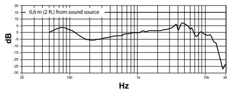
Respuesta de frecuencia típica
