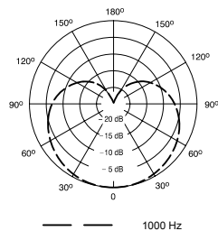
Patrón polar de captación típico
