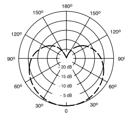
Courbe de directivité typique
