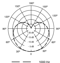
Diagramma polare tipico
