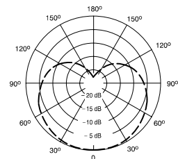
Diagramma polare tipico
