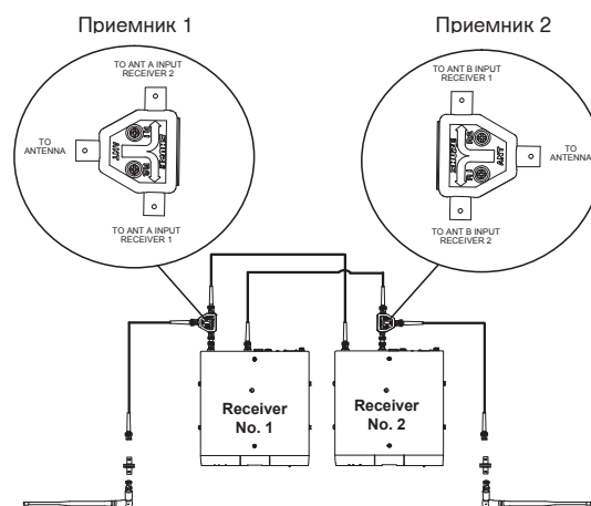
Соединения UA221
