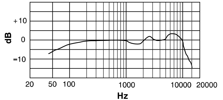
TYPISCHER FREQUENZGANG
