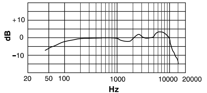
RESPUESTA DE FRECUENCIA TIPICA
